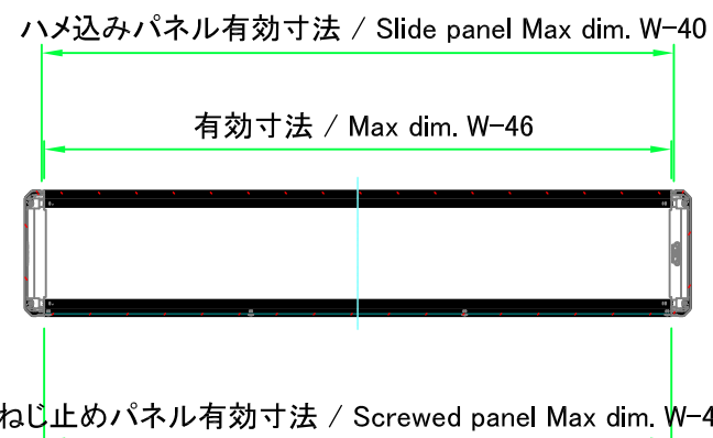
A-A (1:10)
